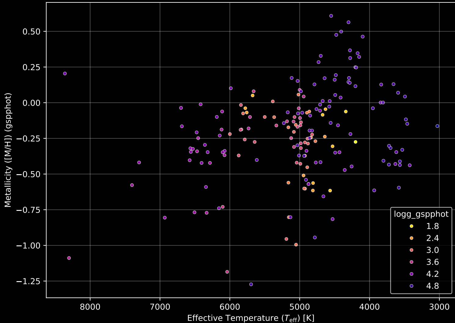
APOGEE DR17 Field: [100+60] Stellar Population Parameters (n= 181)
